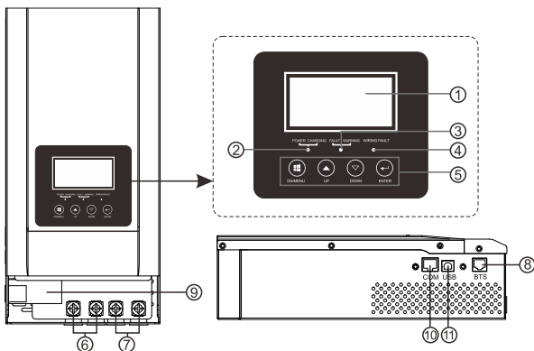
Внешний вид контроллера UB60
